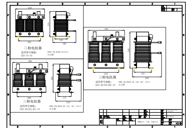
三相调谐电抗器尺寸图
