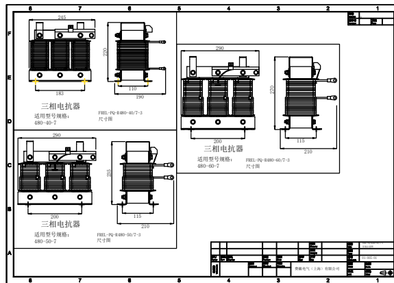
三相调谐电抗器尺寸图2
