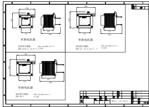
单相调谐电抗器尺寸图1
