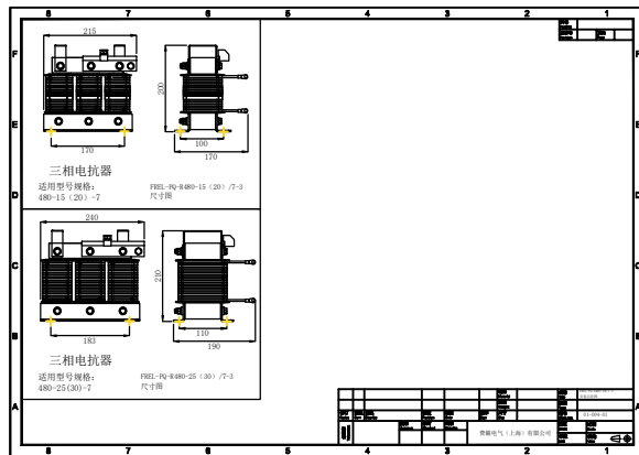
三相调谐电抗器尺寸图1
