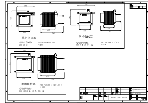
单相调谐电抗器尺寸图2
